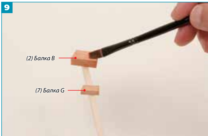
9 Окрасьте балки В и G.
