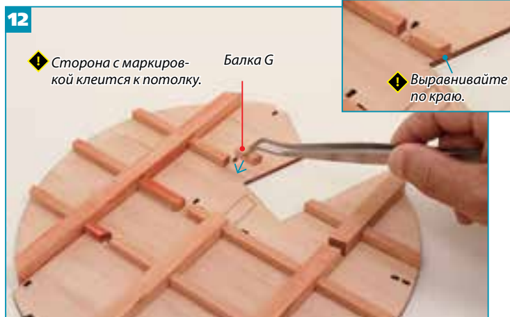
12 Рядом с отверстием для лестницы приклейте балку G.
