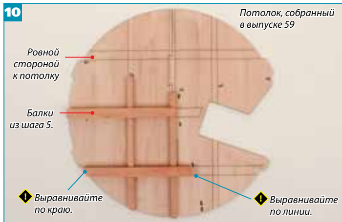
10 Возьмите потолок третьего этажа из выпуска 59 и приклейте к нему балки, собранные в шаге 5.
