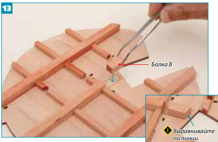
13 Аналогичным образом прикрепите балку В.
