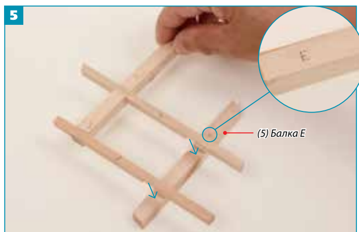
5 В вырезы балок L и J при помощи клея для дерева прикрепите балку E.
